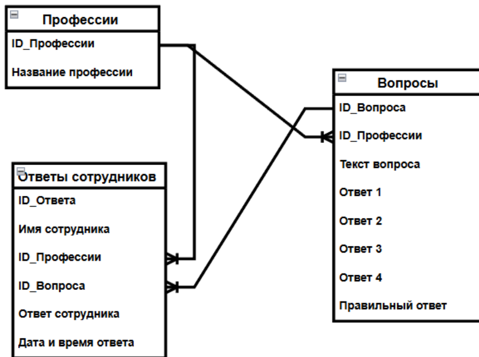
Рисунок 2 - ER-диаграмма структуры хранения данных
